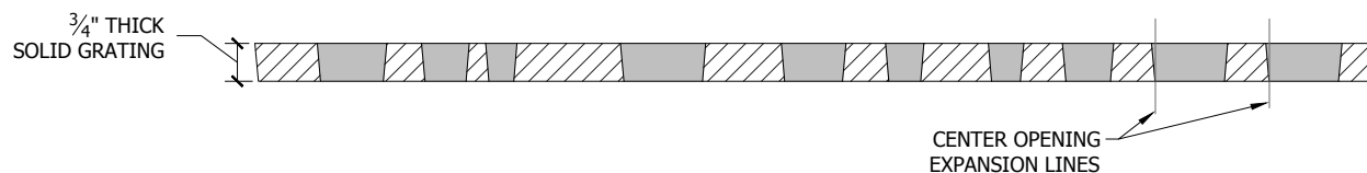
Section A-A'
