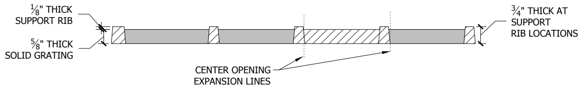
Section A-A'
