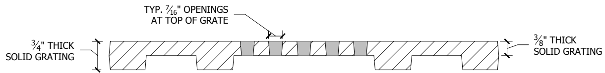
Section A-A'
