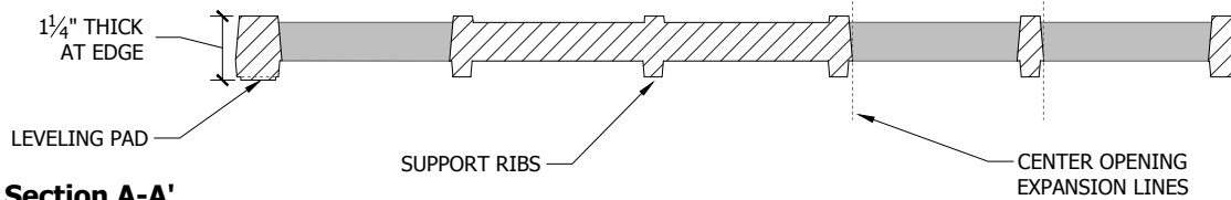
Section A-A'
