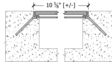
Elevation A-A
