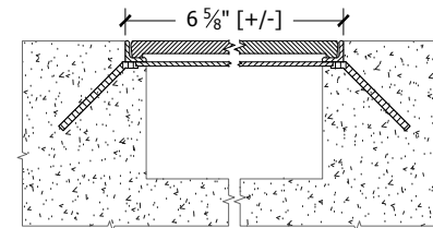
Elevation A-A
