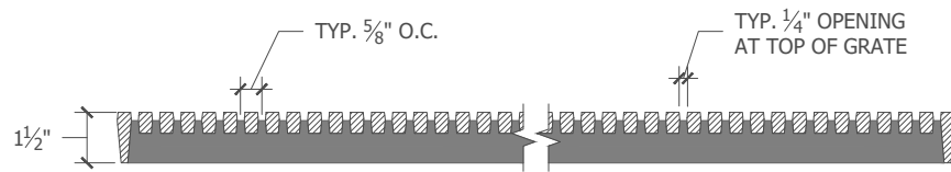
Section A-A'
