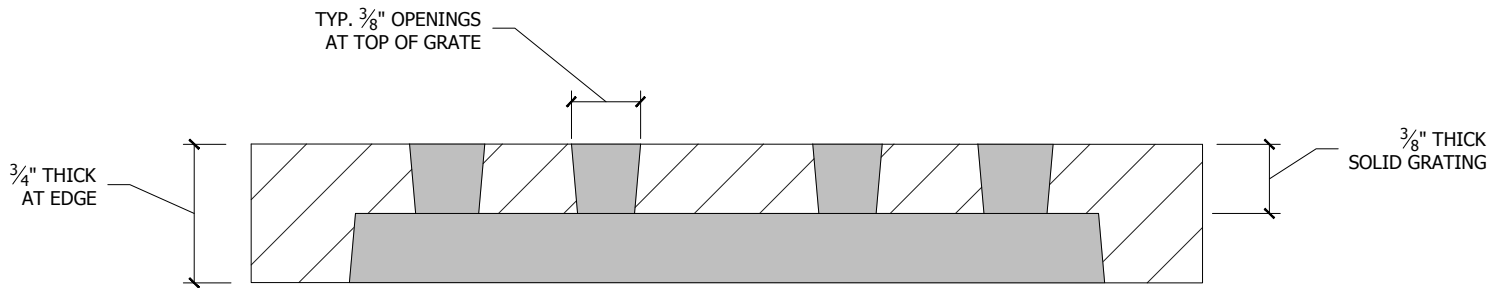
Section A-A'
