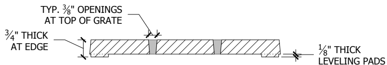
Section A-A'
