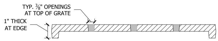
Section A-A'
