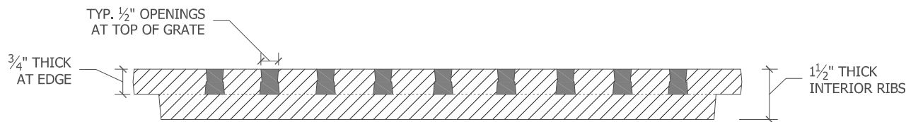
Section A-A'
