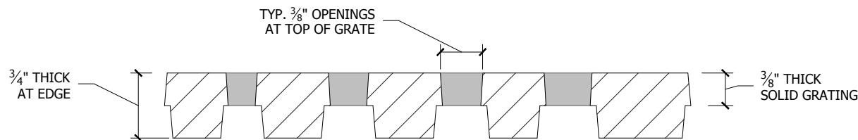
Section A-A'
