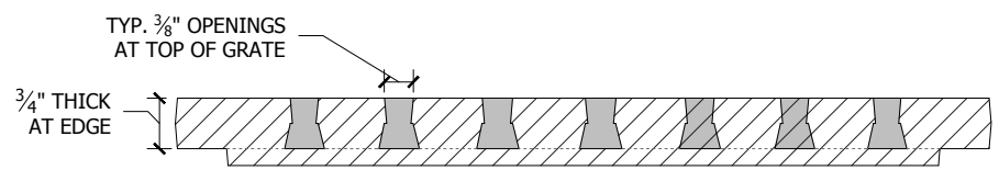
Section A-A'
