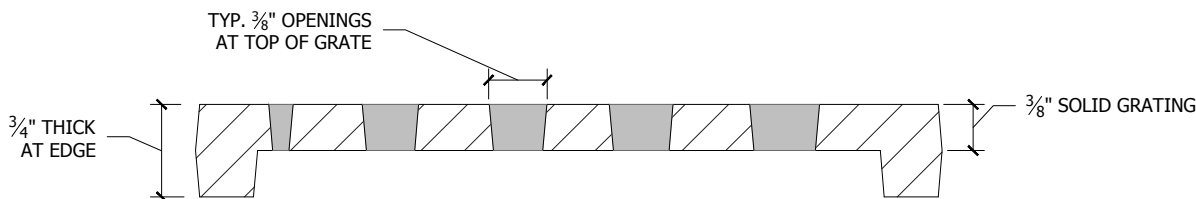
Section A-A'
