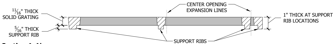
Section A-A'
