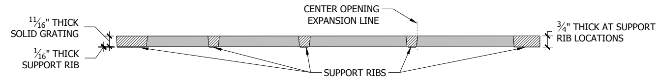
Section A-A'
