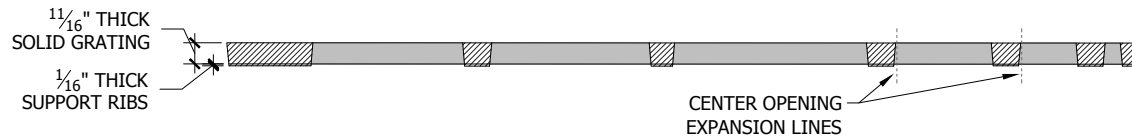
Section A-A'
