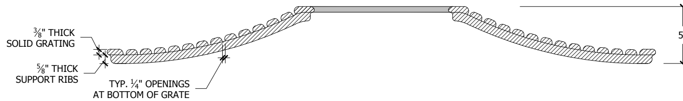
Section A-A'
