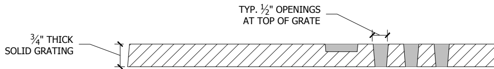
Section A-A'
