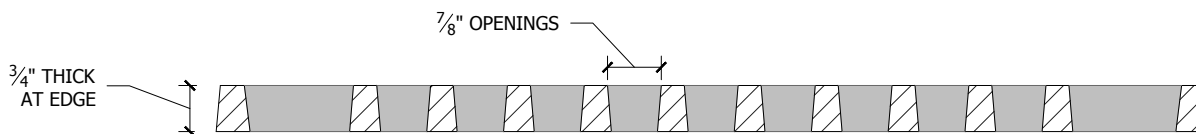
Section A-A'
