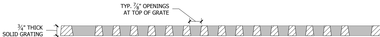
Section A-A'
