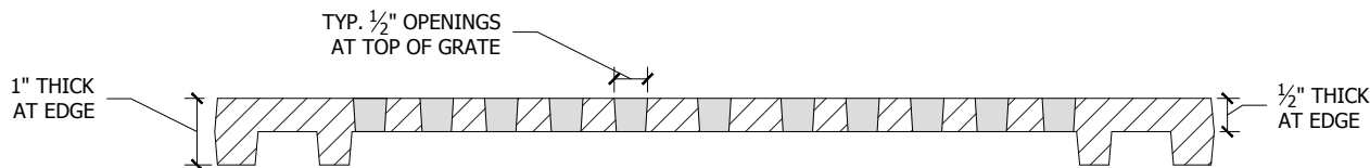
Section A-A'
