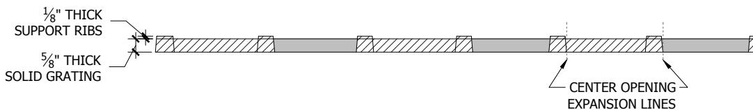
Section A-A'
