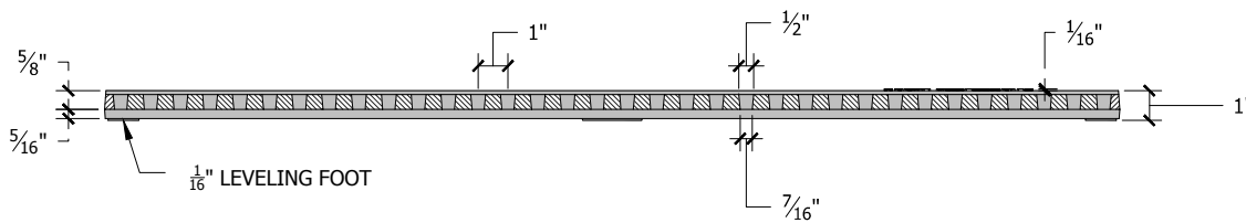
Section A-A'
