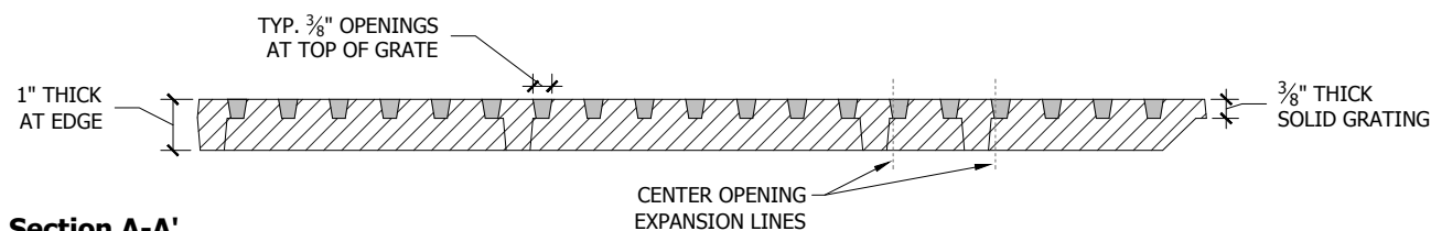
Section A-A'
