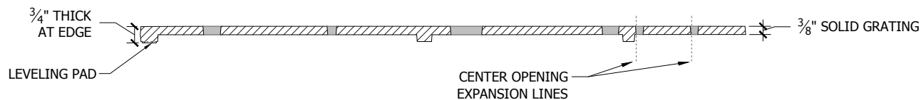
Section A-A'
