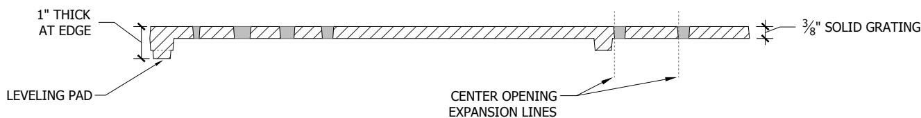
Section A-A'
