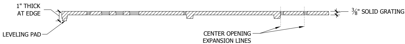
Section A-A'
