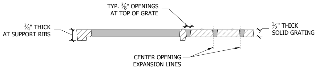
Section A-A'
