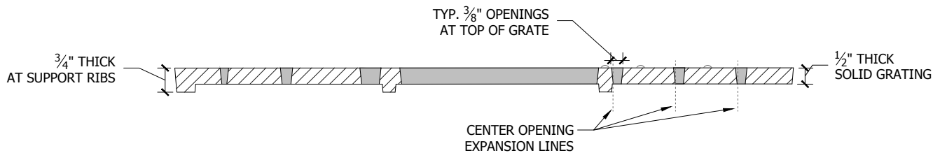
Section A-A'
