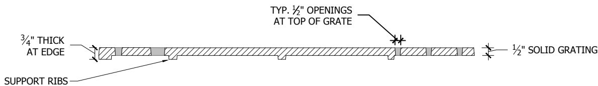
Section A-A'
