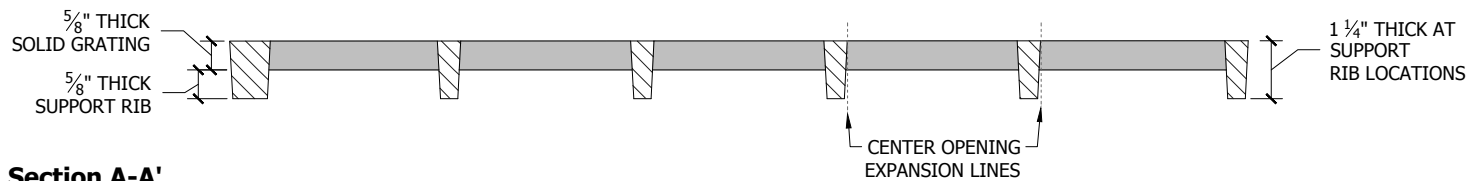
Section A-A'
