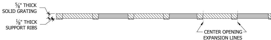
Section A-A'
