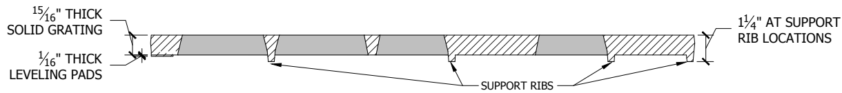
Section A-A'
