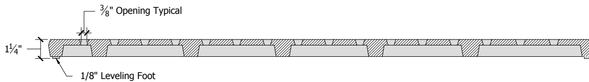
Section A-A'
