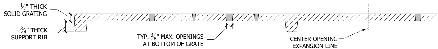
Section A-A'
