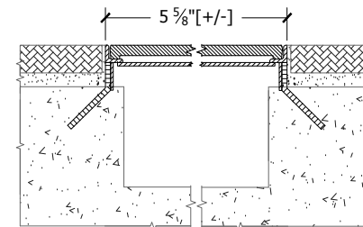
Elevation A-A
