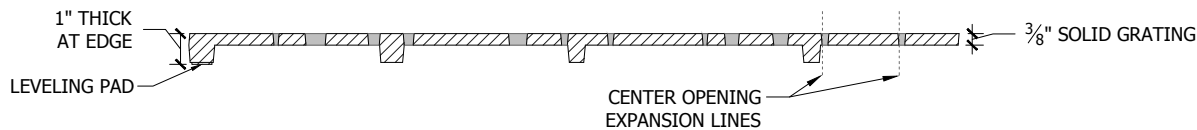
Section A-A'
