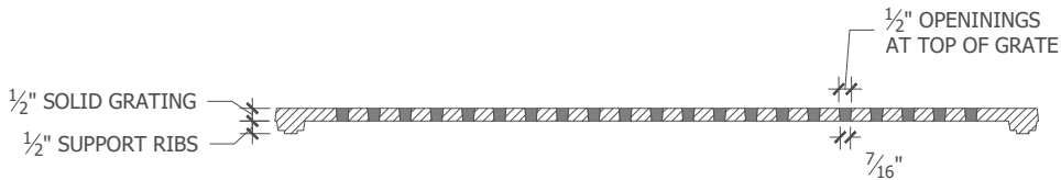
Section A-A'
