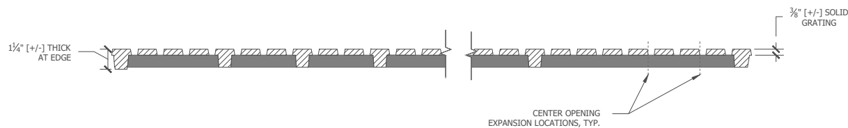
SECTION A-A'
