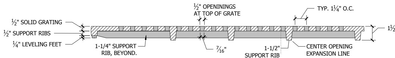
Section A-A'
