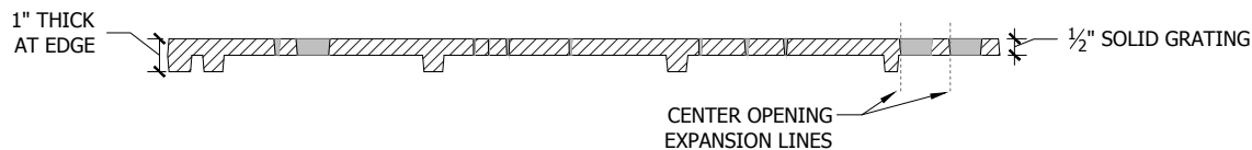
Section A-A'
